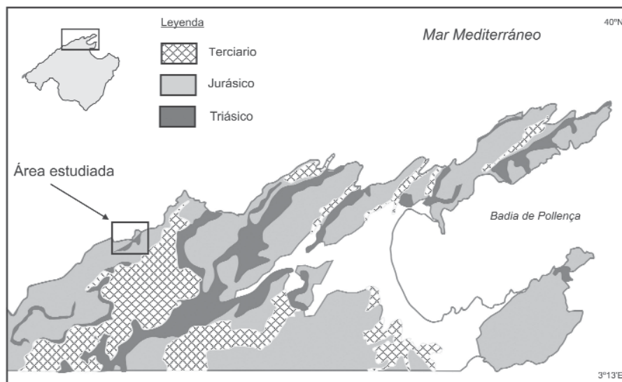
Fig. 1.- Localización geográfica y geológica de las muestras estudiadas. (Mapa modificado de Del Olmo et al. , 1981).
