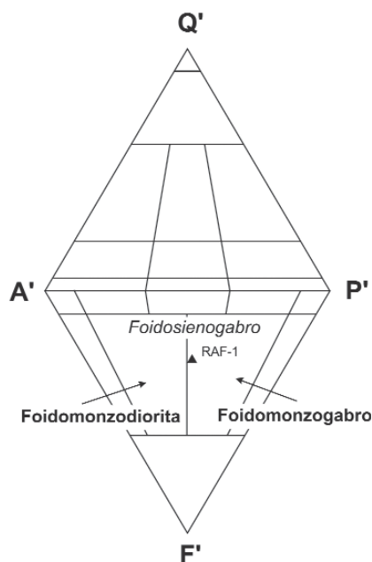
Fig. 3.- Representación de las muestras estudiadas en el diagrama QAPF: Q'A'P'F' son valores normativos.
