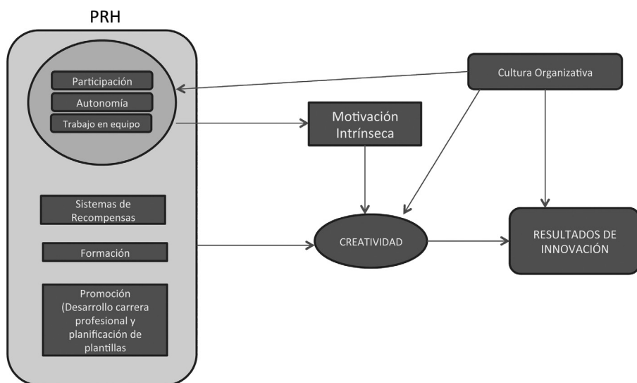
FIGURA 1. MODELO TEÓRICO
