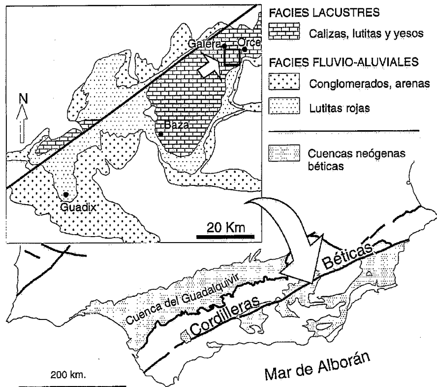
Fig.1.- Esquema geológico de la cuenca de Guadix-Baza (adaptado de García Aguilar y Soria, 1986-87) con indicación del área estudiada.
