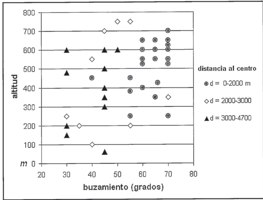
Figura 4: Variación del buzamiento de los diques con la altitud a la que se encuentran. Se han separado los diques en grupos diferentes según la distancia al "centro".
