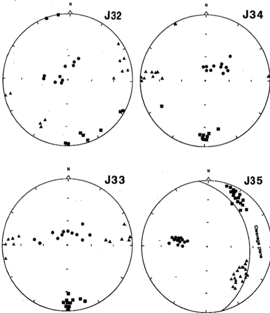
Fig. 2.—Ejes principales de la susceptibilidad magnética máxima (K1, cuadrados), media (K2, triángulos) y mínima (K3, círculos).
