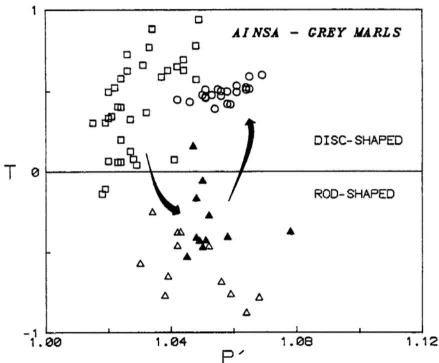
Fig. 3.—Diagrama de anisotropía de Hrouda-Jelinek de las localidades estudiadas: J32 (cuadrados), J33 (triángulos), J34 (triángulos llenos) y J35 (círculos). T-Simetría de la forma del elipsoide, P'-excentricidad del elipsoide.
