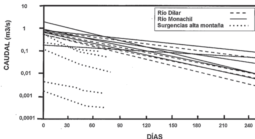
Fig. 3.- Curvas de agotamiento, en escala semilogarítmica, obtenidas para los ríos Dílar y Monachil y para surgencias de la franja glaciaria y periglaciaria
