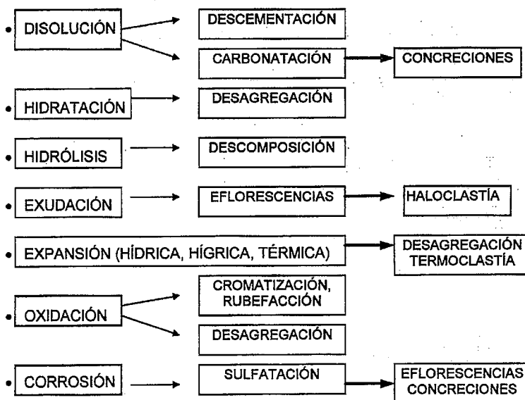
Fig.3.- Esquema de los procesos de alteración de la piedra especialmente relacionados con la naturaleza mineralógica. (Terminología según Ordaz y Eibert, 1988).
