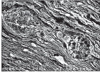
Fig. 2.- Pizarra orgánica de la Fm. Khatatba mostrando orientación preferente de las láminas de arcilla y la presencia de abundantes formas globulares de m.o. reemplazados por pirita y bitumen. Este es también visible rodeando los framboides.
