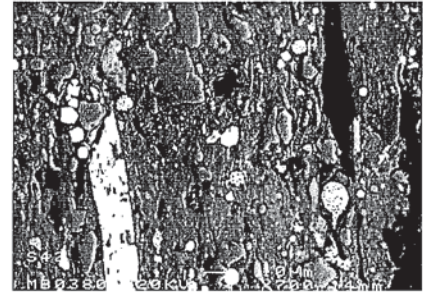
Fig. 4.- Microfábrica de una pizarra orgánica de la Fm. Khatatba. Se observan numerosos granos de cuarzo aleurítico, restos orgánicos piritizados y framboides de pirita. La matriz está formada por una mezcla de m.o. filamentososa y otra masa algal amorfa, donde existen segregaciones de bitumen.
