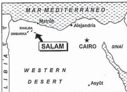
Fig. 1.- Localización del Campo de Salam en el Western Desert (Egipto).
