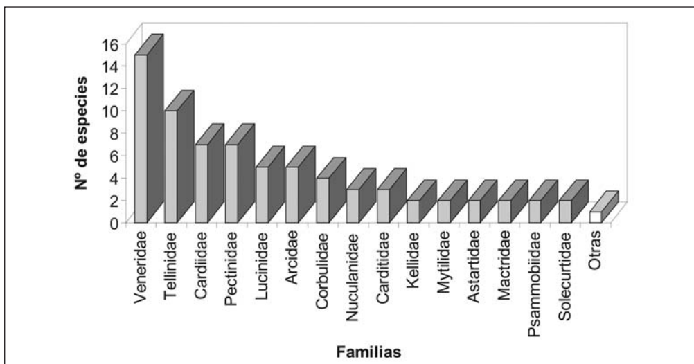
Fig. 3. Representación de las familias de bivalvos del yacimiento de Cacela con mayor diversidad de especies. Fig. 3. Bivalve family histogram from Cacela outcrop with major species diversity.
