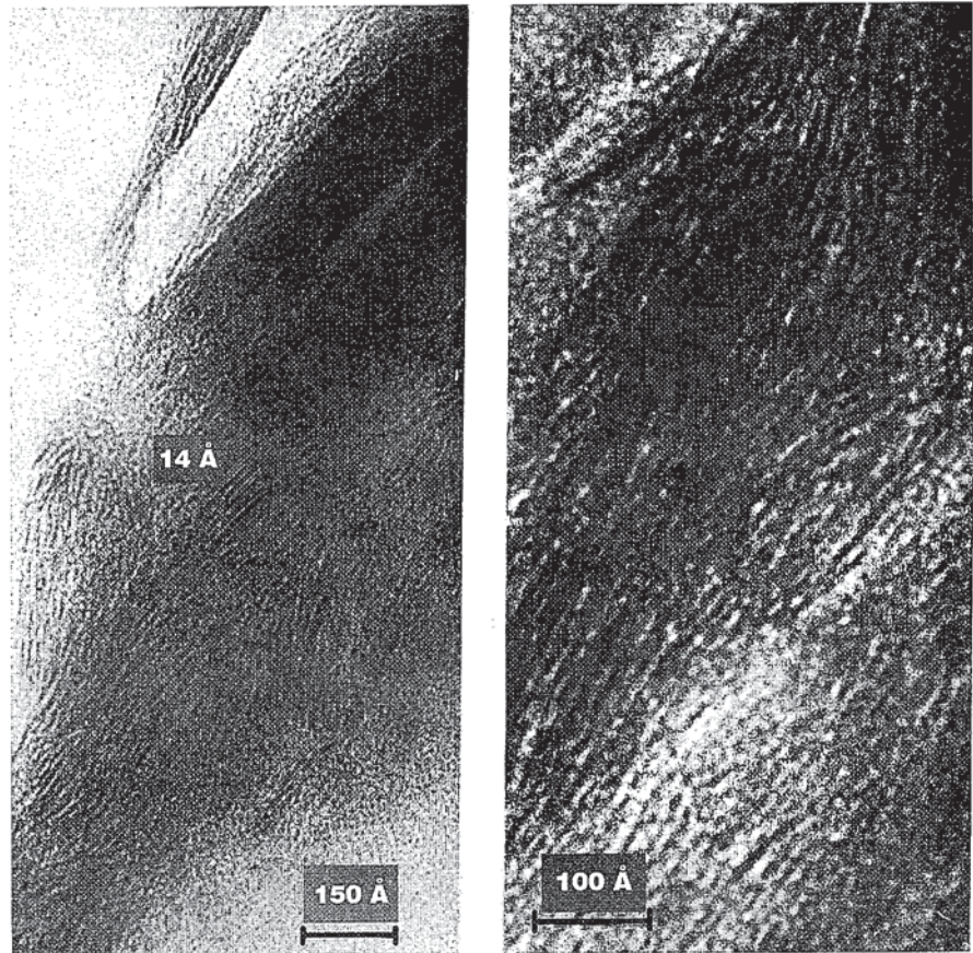
Figura 4: Aspecto de detalle de la muestra SA-AC en MET.
