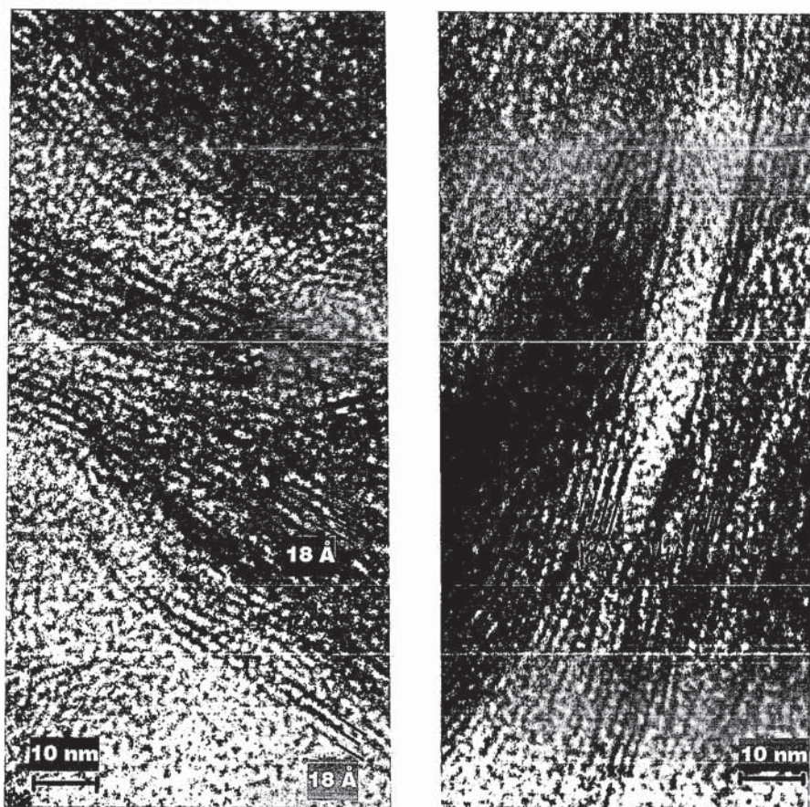
Figura 6: Aspecto de detalle de la muestra SA-PI en MET.
