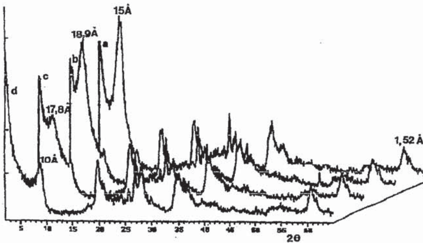
Figura 3: Diagramas de Difracción de Rayos-X de la saponita intercalada, pilarizada y calcinada.
