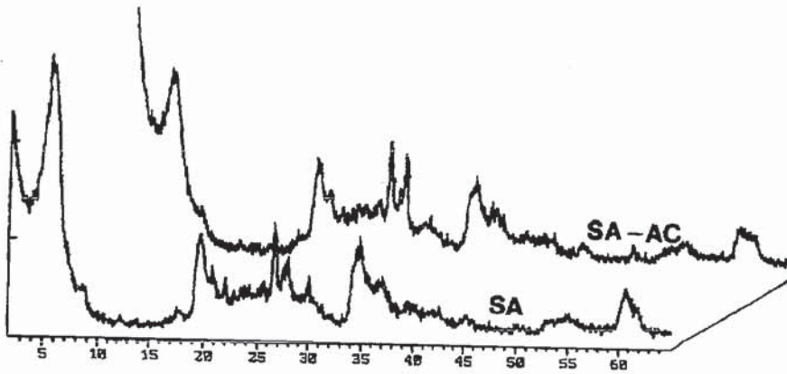
Figura 2: Diagramas de Difracción de Rayos-X de la saponita natural y activada con ácido.
