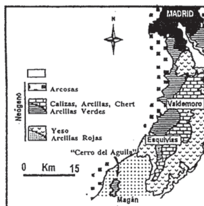
Figura 1: Situación geográfica del "Cerro del Aguila" y esquema geológico.
