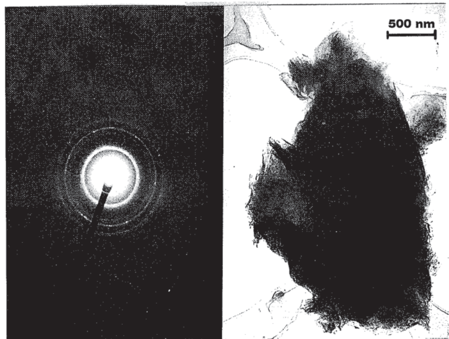
Figura 5: Diagrama de difracción de electrones correspondiente a la muestra SA-AC y partícula analizada.
