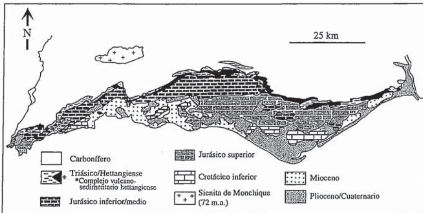
Fig. 3- Esquema geológico de la Cuenca del Algarve
