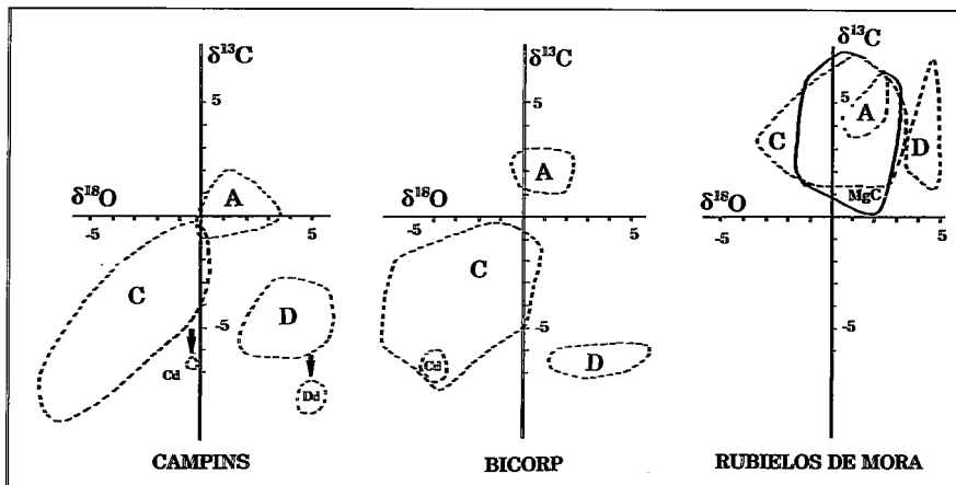
Fig. 2.— Diagramas \delta^{13}\text{C} - \delta^{18}\text{O} de los carbonatos de las cuencas de Campins, Bicornp y Rubielos de Mora. Carbonatos primarios: A aragonito, C calcita, D dolomita, MgC calcita magnesiana. Carbonatos diagenéticos: Cd calcita diagenética, Dd dolomita diagenética. Las flechas indican la incorporación de \text{CO}_2 ligero en los minerales diagenéticos.
