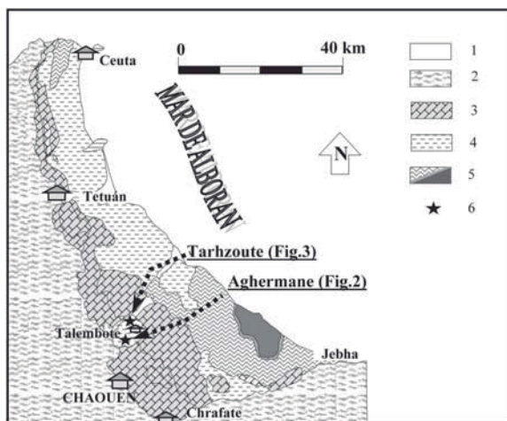
Fig. 1.- Mapa geológico simplificado del Rif septentrional modificado de Suter, (1980) con la localización de los dos afloramientos del Paleógeno inferior de la cobertera gomáride. 1: Plio-Cuaternario, 2: Zona Externa y unidades de los Flyschs, 3: Dorsal Caliza y grupo de Jebel Musa, 4: Unidades gomárides y su cobertera eocena-miocena, 5: Sébtides, 6: localización en el mapa de los afloramientos estudiados.
