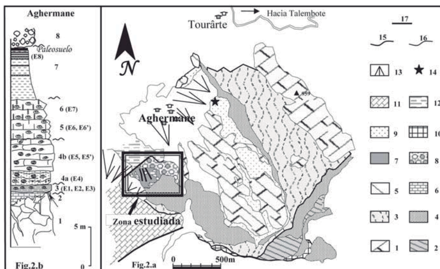
Fig. 2.- 2a: Mapa geológico simplificado de la zona de Aghermene mostrando la localización de los afloramientos del Eoceno-Mioceno Inferior del manto paleozoico gomáride superior de Talembote, 1: Calizas con Favosites del Devónico inferior de la unidad superior de Talembote, 2: Devono-carbonífero del manto de Koudiat Tiziane en Talembote, 3: Grauwackas en grandes bancos y filitas oscuras del Carbonífero del manto de Talembote, 4: Facies Verrucano del Permo-Trias, 5: Calizas masivas blancas (C.M.B) del Lías inferior, 6: Calizas con Alveolinas y Assilinas del Eoceno Inferior-medio, 7: Margas amarillentas de la base del Bartonense, 8: Conglomerado poligénico del Mioceno Inferior, 9: Pelitas con bancos finos de areniscas (facies de tipo Viñuela) del Burdigaliense inferior, 10: C.M.B del Lías de las escamas de Ouaslaf (Dorsal interna), 11: Formaciones carbonatadas del Triás-Lías de la Unidad de Jebel Tissouka (Dorsal externa), 12: Areniscas y pelitas marrones del Mioceno Inferior de la predorsal, 13: Derrubios y formaciones aluviales cuaternarias, 14: Sedimentos de tipo Viñuela datados del Burdigaliense inferior mediante foraminíferos planctónicos, 15: contacto normal, 16: Contacto anormal, 17: Fallas. 2b: Columna litoestratigráfica de la serie eocena-miocena de Aghermene.
