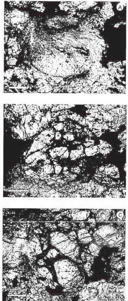
Fig. 1.- Cóndrulos seleccionados en Reliegos. Todas las fotos se han realizado con luz transmitida y nicoles paralelos. A) REL 3. Cóndrulo radial de piroxeno, formado por acículas muy finas. B) REL 2. Cóndrulo porfídico de olivino, flanqueado por granos metálicos, que se ven oscuros. C) REL 4. Cóndrulo porfídico de olivino, con mesostasia abundante entre los cristales.
