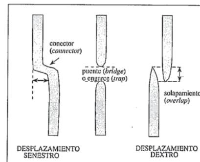
Fig. 6.- Terminología para el desplazamiento de un dique en sección plana. Adaptado de Rickwood (1990).
