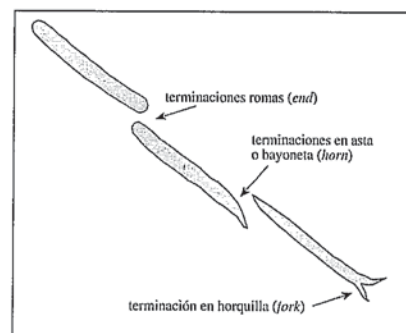
Fig. 7.- Segmentos de un dique en sección plana mostrando terminaciones romas, en asta y en horquilla. Adaptado de Rickwood (1990).
