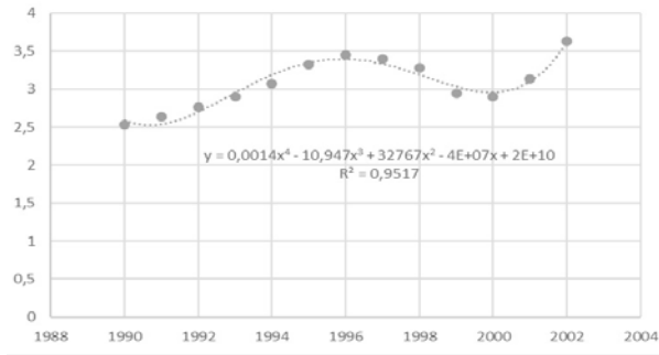
FIGURA 5.3.1. OIP (INCLUYENDO OXIGENO), EN PETAGRAMOS (1990-2002)
