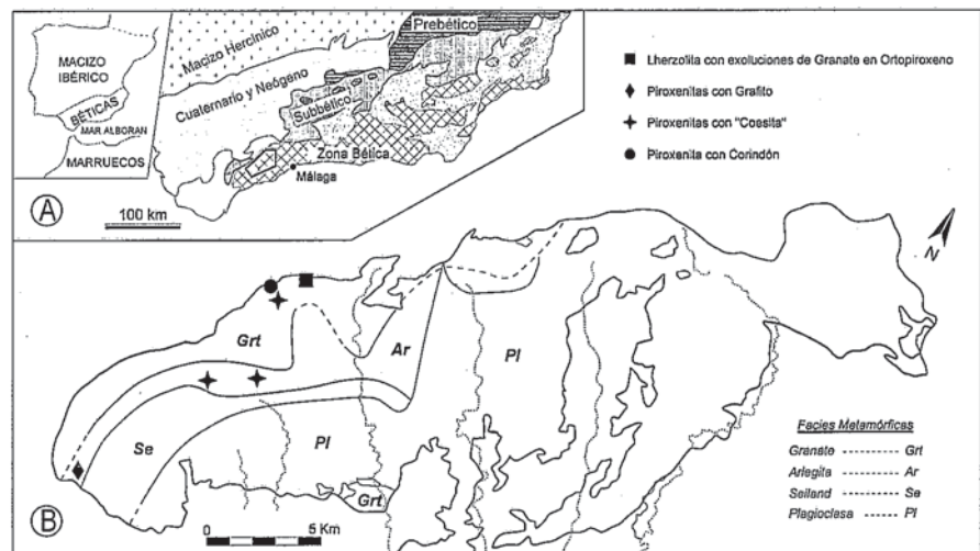
Fig. 1.- A: Mapa esquemático de las Cordilleras Béticas. El recuadro dibujado al oeste de Málaga señala la localización del macizo de peridotitas de Sierra Bermeja. B: Zonación petrográfica del Macizo de Sierra Bermeja, según Obata (1980), en el que se muestra la procedencia de las muestras con evidencias de metamorfismo de alta o ultra-alta presión.
