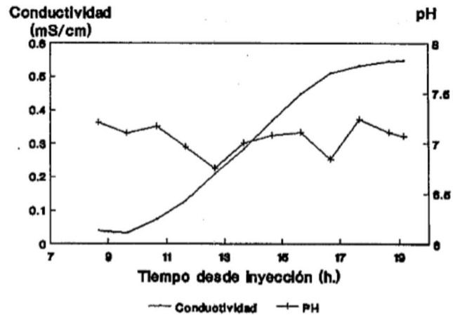
Fig. 2.— Evolución del pH y de la conductividad durante la segunda experiencia.
