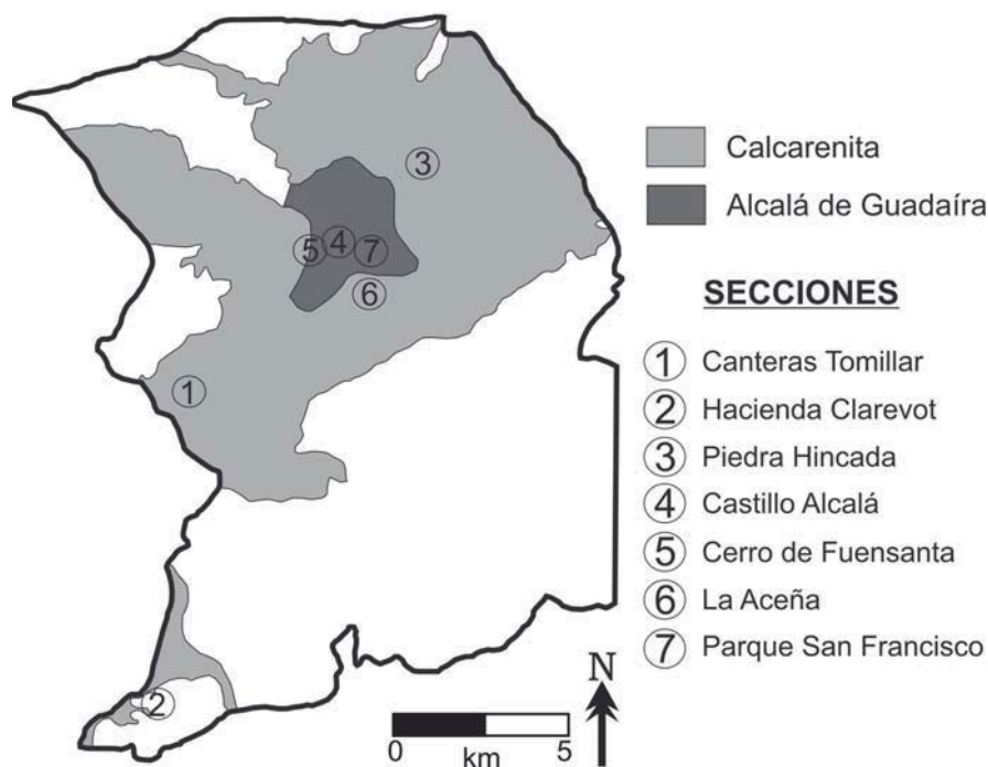
Fig. 1.- Localización de las secciones estratigráficas y distribución de las calcarenitas messinienses en el área de Alcalá de Guadaira (Sevilla, SO España).
