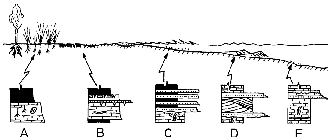
Fig. 2.—Modelo de sedimentación y distribución de secuencias.
