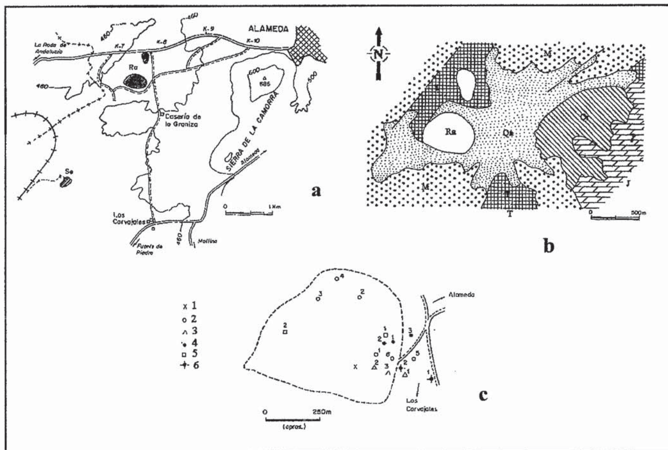
Fig. 1.- a: Localización de la laguna de la Ratoso (Ra) y topografía del área, incluyendo la situación de otras zonas inundables próximas. b: Esquema geológico (Martín Serrano, 1986). T: Trías, J: Jurásico, M: Mioceno, Qr: Depósitos de vertiente (Cuaternario), Qa: Depósitos aluviales (Cuaternario). c: Situación de los diferentes puntos de adquisición de datos. 1: Escala limnimétrica, 2: Muestras superficiales, 3: Infiltrometrías, 4: Sondeos hincados, 5: Catas, 6: Sondeos mecánicos.
