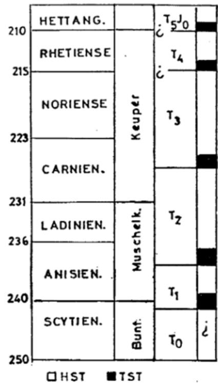
Fig. 2.- ( T_1 a T_4 ): Secuencias de Depósito diferenciadas. ( T_0 ): Supersecuencia tipo rift. (?) Límite cronoestratigráfico y contenido secuencial desconocido.
