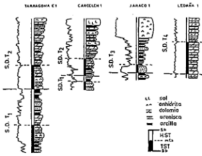
Fig. 4.- Ejemplos de interpretación en System Tracts.
