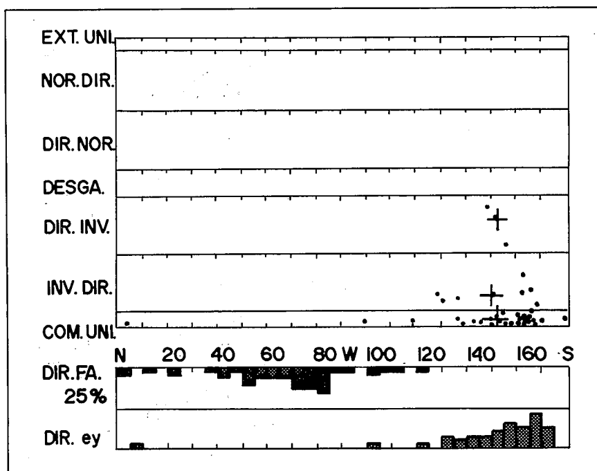
Fig. 1.—Relaciones de los tipos de fallas con la dirección del máximo acortamiento horizontal (0-180) K'/\text{dirección } e, K'=e_x/e_z . Deducido de las fallas pertenecientes a la etapa Guadarrama en la zona estudiada (puntos). Los valores medios para cada tipo de fallas (cruces) dan direcciones de acortamiento próximas a N150E. En la parte inferior se representan dos histogramas, el superior correspondientes a las direcciones de fallas activas (0-180) y el inferior a las direcciones de compresión para cada falla (De Vicente, 1988) de esta fase.
