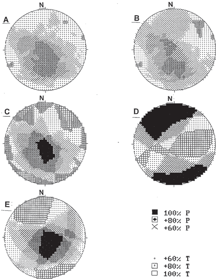
Fig. 3- Diagramas de diedros rectos de los mecanismos focales de los sismos de la serie Agrón. Proyección estereográfica, hemisferio inferior. A, todos los sismos (38 datos). B, sismos con m>2.5 (11 datos). C, mecanismos de falla normal y m>2.5 (8 sismos). D, mecanismos de falla inversa y m>2.5 (3 sismos). E, sismos con m≤2.5 (11 datos). Programa, G. de Vicente.
