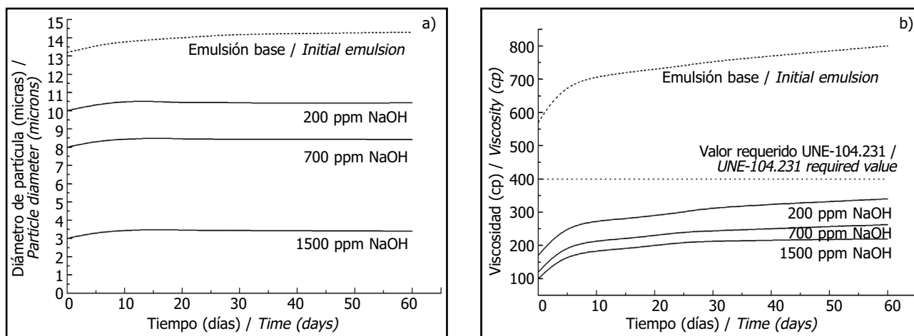
Figura 2. Evolución con el tiempo de las emulsiones con NaOH: a) tamaño de partícula, b) viscosidades. Figure 2. Variation in NaOH-containing emulsions: a) mean particle size, b) viscosity.
