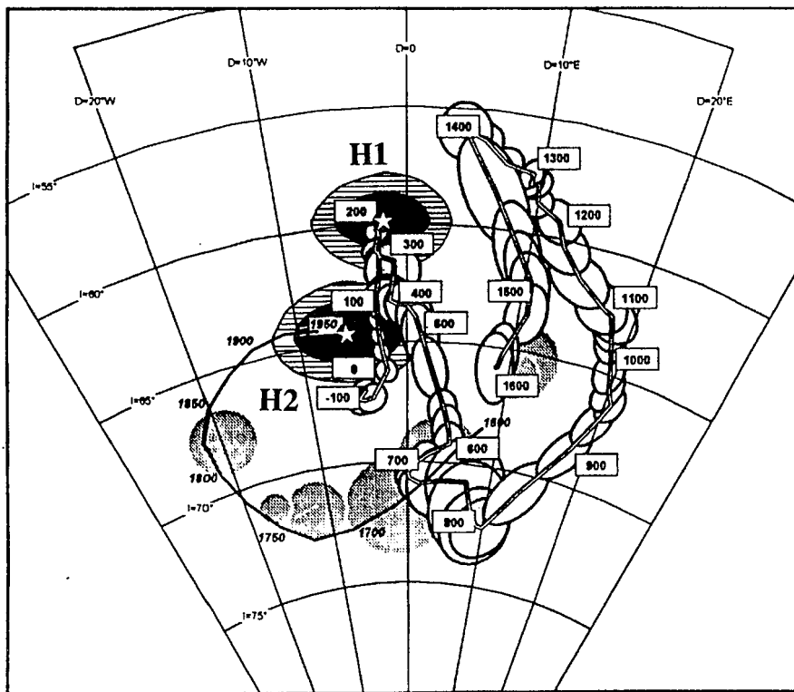
Fig. 3.- Curva de variación secular del Campo Magnético Terrestre de los últimos 2100 años establecida para París por Bucur (1994). H1 y H2 representan las direcciones medias (estrellas blancas) con su error estadístico en negro, y el debido a la corrección CVP sombreado.
