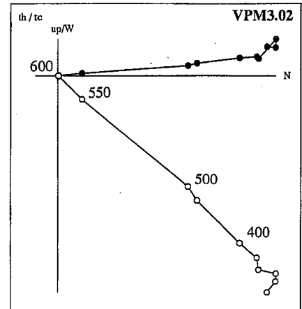
Fig. 1.- Proyección ortogonal de la desimación térmica de la NRM en coordenadas geográficas de una muestra representativa. Los círculos negros son proyecciones sobre el plano horizontal y los blancos sobre el vertical. Los números sobre las curvas están en grados centígrados.
