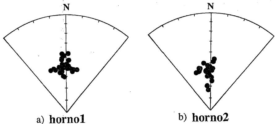
Fig. 2.- Distribución de las direcciones obtenidas para las muestras sobre un diagrama polar en coordenadas geográficas, que representa la declinación (D) sobre el arco, y la inclinación (I) sobre el radio. a) direcciones de las muestras del horno 1. b) direcciones de las muestras del horno 2.
