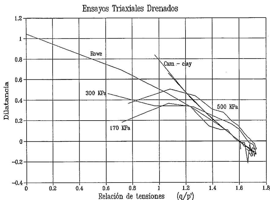
Fig. 2.- Medidas de dilatancia obtenidas a partir de los resultados de los ensayos triaxiales CD. Fig. 2.- Dilatancy measures obtained from the triaxial CD tests.
