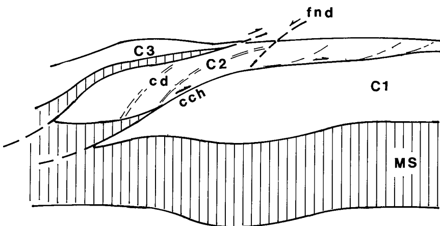
Fig. 4.—Acortamiento asimétrico de la litosfera previamente estirada, según el modelo de la figura 3. MS: Manto superior litosférico. cch: Cabalgamiento cortical hercínico. fnd: Fallas normales dúctiles. cd: Cizallas dúctiles.
