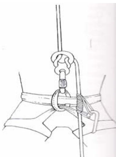
Dibujo nº11 .- Rapelando con autoseguro mediante un nudo, el marchand (fuente: Murcia, 1996)
