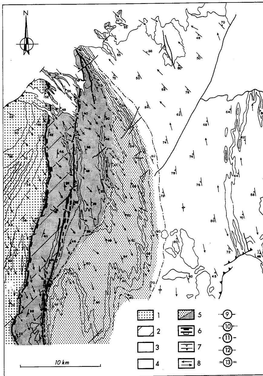
Fig. 1. Mapa estructural y metamórfico del sector de Somosierra del Sistema Central Español. Dominio occidental: (1) Gneises de alto grado y migmatitas. Dominio oriental: (2) Micaesquistos con St+Sil\pm Ky de grado medio (zona de la sillimanita); (3) pizarras y cuarzoesquistos de grado bajo a medio (zona clorita-biotita a estaurólita). (4) Rocas Mesozoicas y Cenozoicas. (5) Zonas de deformación: zona de crenulación superior (punteado) y milonitas S-C (punteado suave). (6) «Detachments» de bajo grado con zonas ultramiloníticas y filoníticas: (relleno negro) de Montejo y (relleno blanco) del Cervunal. (7) Dirección y buzamiento de la esquistosidad S1 (relleno blanco) y de la foliación milonítica S2 (relleno negro). (8) Lineaciones: (flecha superior) lineación de intersección L1, (flecha inferior) lineación mineral y/o de estiramiento L2, con indicación del movimiento del bloque superior. Isogradas minerales: (9) cloritoide (+); (10) granate (+), (11) estaurólita (+); (12) sillimanita (+) y (13) andalucita (+).
