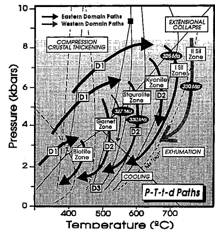
Fig. 3. Trayectorias P-T-t de los diferentes niveles estructurales del dominio oriental y occidental. D1 y D2 son los principales eventos tectonotérmicos. D3 representa los eventos deformativos tardíos. Las líneas continuas y discontinuas representan los equilibrios de la Fig. 2. «Ms out»: Ms+Pl+Qtz=Sil+Kfs+L (Vielzeuf, D. & Holloway, 1988).
