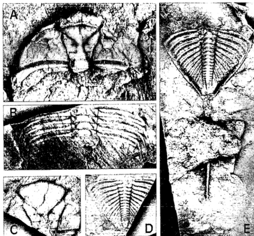
Fig. 1.- Preodontochile batalleri (Hernández Sampelayo), Telychiense, Corral de Calatrava (Ciudad Real). A, réplica en látex del cefalón MGM-744-S (x 3,2); B, idem. de cuatro segmentos torácicos, MGM-746-S (x 3); C, idem. del cráneo MGM-745-S (x 3); D, molde interno de un fragmento pigidial, MGM-747-S (x 2); E, réplica en látex de un pigidio completo, MGM-748-S (x 2,5).
