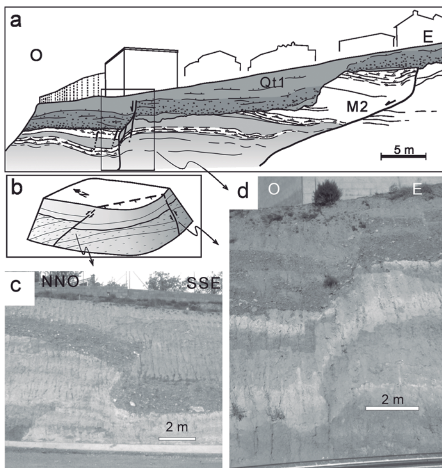
Fig. 3.- Deformación de la terraza inferior 2 km al norte de Teruel (ver Fig. 1). (a) Corte general, M1 Mioceno superior, Qt1 terraza baja, (b) esquema 3-D de la falla post-terrace inferior en relación con los dos taludes que la cortan, (c) y (d) aspecto de dicha falla en ambos taludes.
