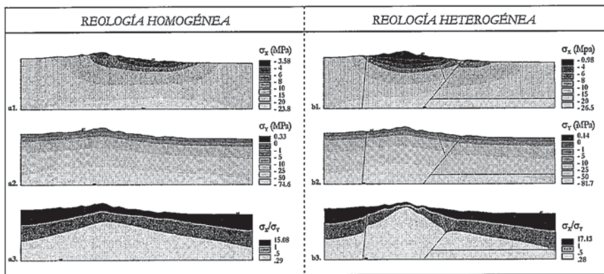
Fig.3.- Diagramas de contornos de la distribución de esfuerzos al aplicar la gravedad y una carga horizontal de 20 MPa (a. reología homogénea y b. variaciones litológicas): a1-b1. magnitudes de s_x (megapascales), a2-b2. magnitudes de s_y (megapascales) y a3-b3. magnitudes de s_x/s_y . Las representaciones se han limitado hasta una cota de -2000 m. Los valores de esfuerzos negativos indican compresión y los positivos extensión. En cuanto al factor de forma, los valores positivos implican que s_x y s_y tienen igual signo, y las magnitudes menores y mayores que 1 indican respectivamente que s_y > s_x o s_x > s_y . MX, localización del valor máximo, y MN, localización de valor mínimo.
