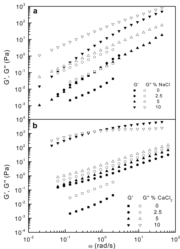
Figura 2 Evolución de las funciones viscoelásticas lineales de las dispersiones de yema con un contenido del 45% (p/p) en sólidos a) influencia de la concentración de NaCl, b) influencia de la concentración de \text{CaCl}_2 .
