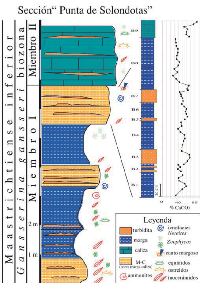
Fig. 2.- Variaciones del (%) \text{CaCO}_3 en margas con celestita y turbiditas.
