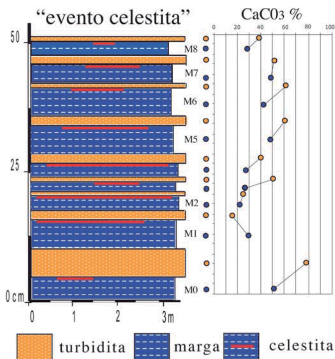
Fig. 2.- Variaciones del (%) \text{CaCO}_3 en margas con celestita y turbiditas.
