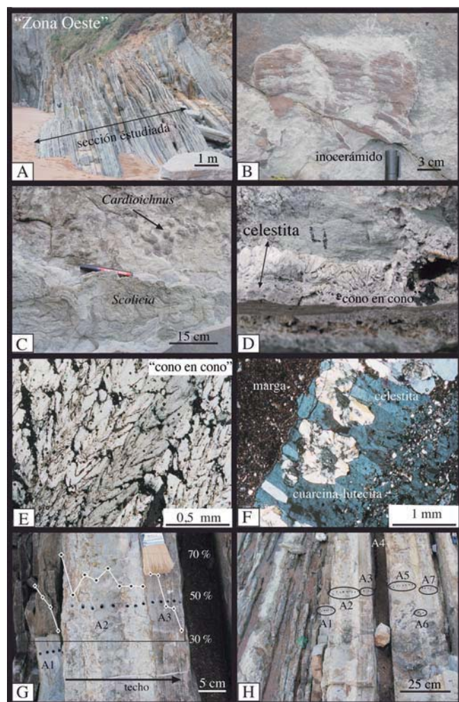
Fig. 4.- Diferentes imágenes de la sección de «Sopelana Oeste».
