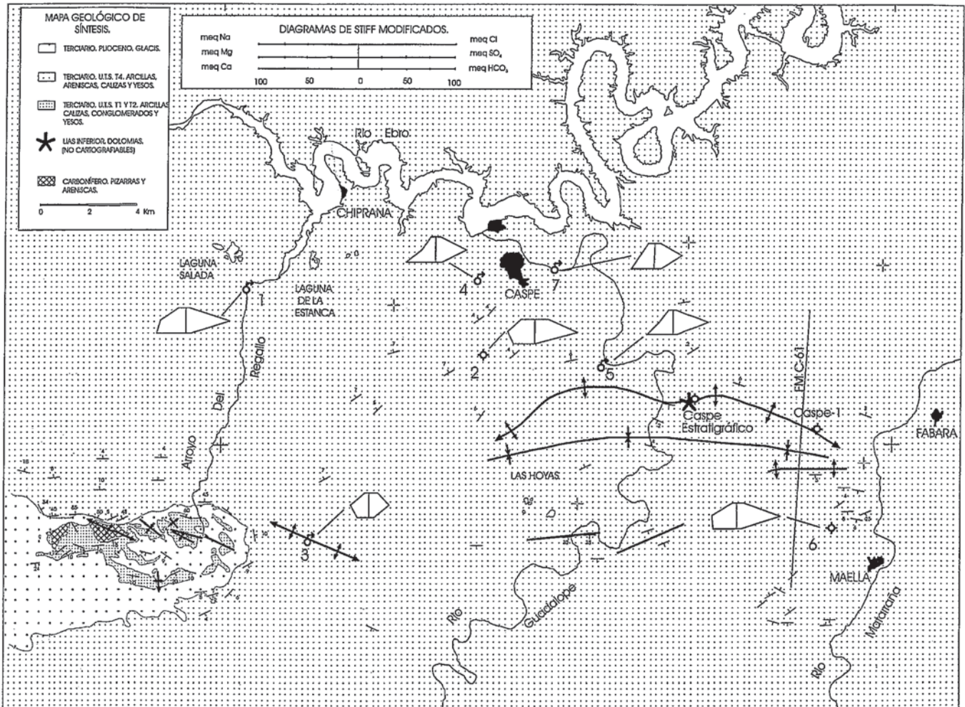
Fig. 2- Mapa geológico de síntesis (basado en IGME, 1981; Medial de Vega, 1969 y Villena et al, 1992 y datos propios) y diagramas de Stiff modificados. Fig. 2- Geological map of synthesis (based on IGME, 1981; Medial de Vega, 1969 and Villena et al, 1992 and own dates) and diagrams of modified Stiff.
