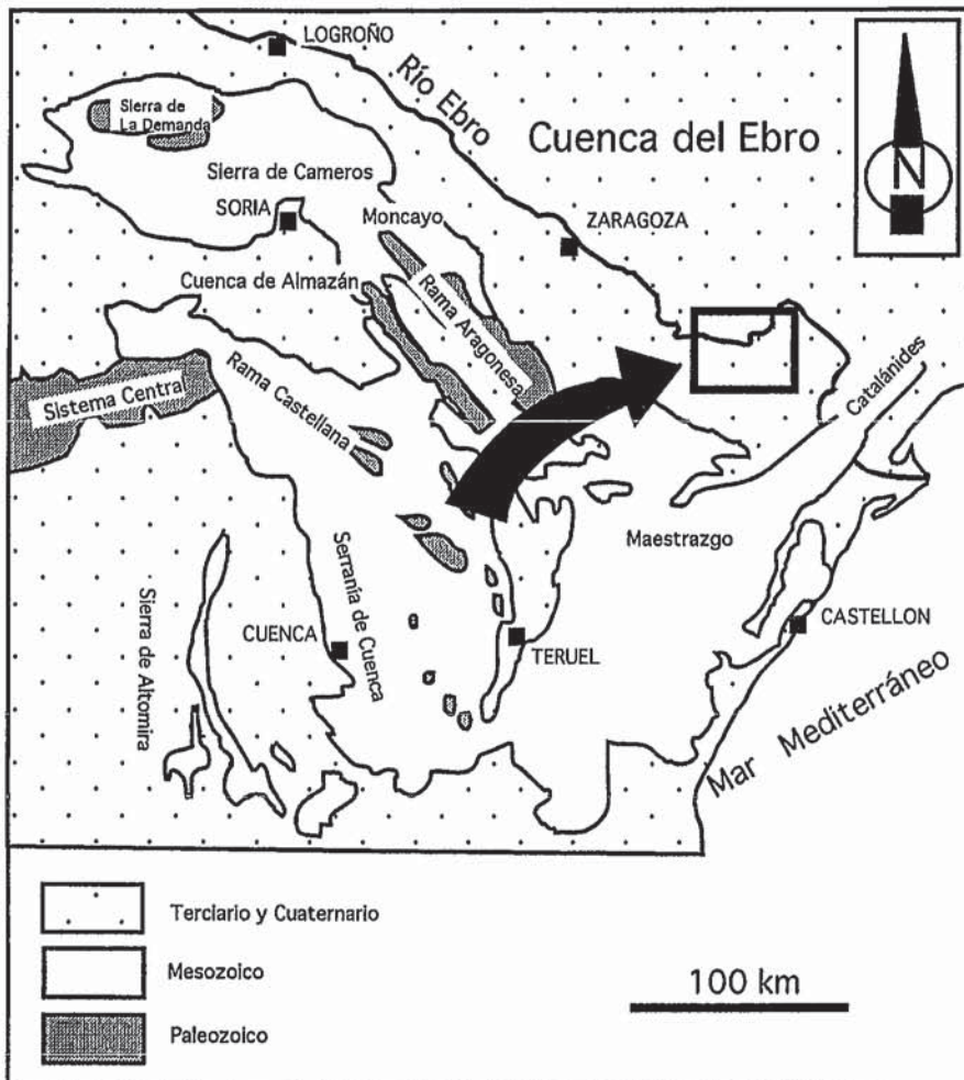
Fig. 1- Situación geológica
