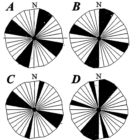
Fig. 3.- Resultados generales (A) para el total de las 24 sub-imágenes; y parciales (B, C y D) en función de las distintas comarcas: Llanura Manchega, Campo de Montiel y Campo de Calatrava, respectivamente.
