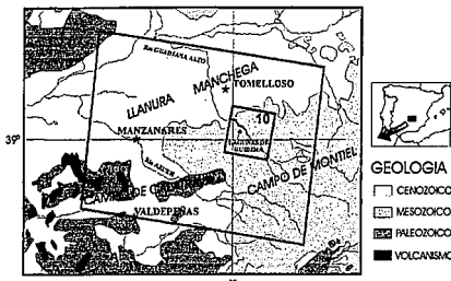
Fig. 1.- Esquema geológico general (I.G.N., 1992); situación de las unidades fisiográficas principales; situación del área estudiada mediante imágenes LANDSAT (ventana ejemplo resaltada).
