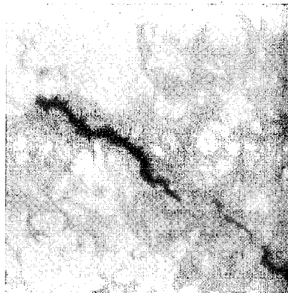
Fig. 3.- Resultados generales (A) para el total de las 24 sub-imágenes; y parciales (B, C y D) en función de las distintas comarcas: Llanura Manchega, Campo de Montiel y Campo de Calatrava, respectivamente.
