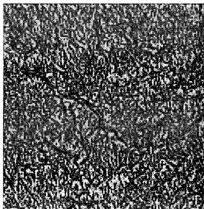
Fig. 2.- Ejemplo del procesado en una de las veinticuatro ventanas (Lagunas de Ruidera).
