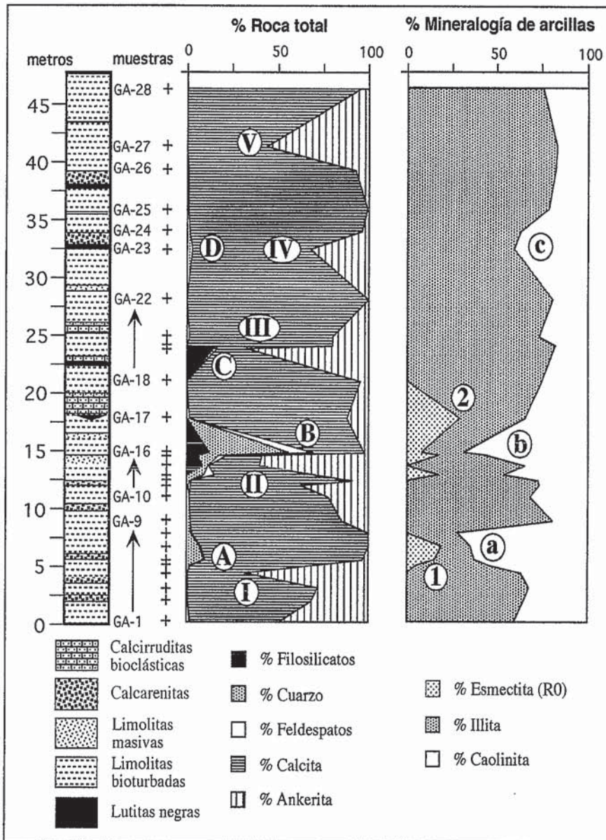
Fig.1.- Sección estratigráfica y composición mineralógica de la Formación de Quintanaloma en Gredilla de Sedano. Se detectan cuatro eventos terrígenos principales (A, B, C, D); cinco de precipitación de ankerita (I, II, III, IV, V); dos de illita (1, 2) y tres de caolinita (a, b, c).
