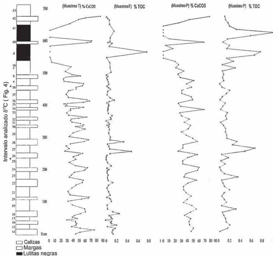
Fig. 2.- Serie de detalle y curvas de contenido en CaCO 3 y carbono orgánico (TOC) para el intervalo analizado (biozona tenuicostatum ). Muestreo T a tiempo constante y muestreo P a potencia constante (explicación en el texto). Se muestra la numeración de las capas marcadas en el campo.
