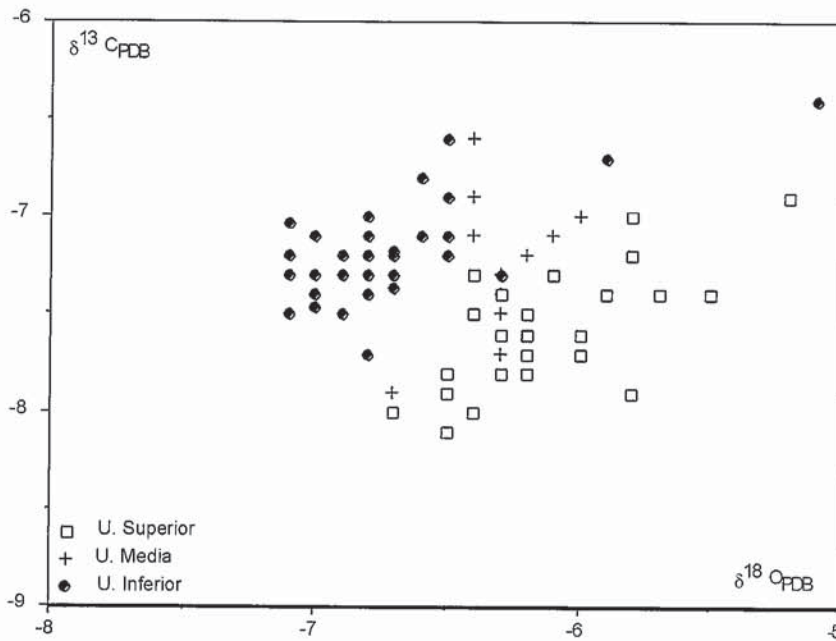
Fig. 3.- Diagrama \delta^{13}C_{PDB} versus \delta^{18}O_{PDB} correspondiente a las calizas palustres de la sucesión miocena en la región suroriental de la Cuenca del Duero. Nótese la moderada correlación de los puntos de la U. Superior ( r = 0,69 ; n = 27 ).
