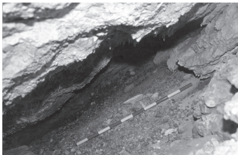
Lám. 22: Sector II. Detalle. Sedimentos con restos óseos de fauna sellados por placa estalagmítica.
