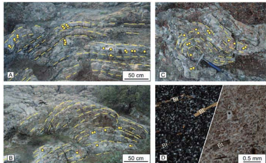
Fig. 2. A, B, C) Aspecto de campo de las estaciones muestreadas (CR-1, CR-2 y CR-3 respectivamente) para el análisis de la anisotropía de la susceptibilidad magnética. Los puntos representan la localización de algunas muestras perforadas y las líneas discontinuas, las trazas del bandeo magmático. D) Microfotografías mostrando el aspecto de la matriz microcristalina de una de las muestras: nicols cruzados (izquierda) y paralelos (derecha). Obsérvese la orientación preferente de los fenocristales de biotita (Bt). Ver figura en color en la web.
