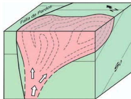
Fig. 5. Reconstrucción tridimensional de la intrusión de Cerro Redondo con indicación de la dirección de flujo ígneo (flechas blancas). So: estratificación del encajante paleozoico. Ver figura en color en la web.
