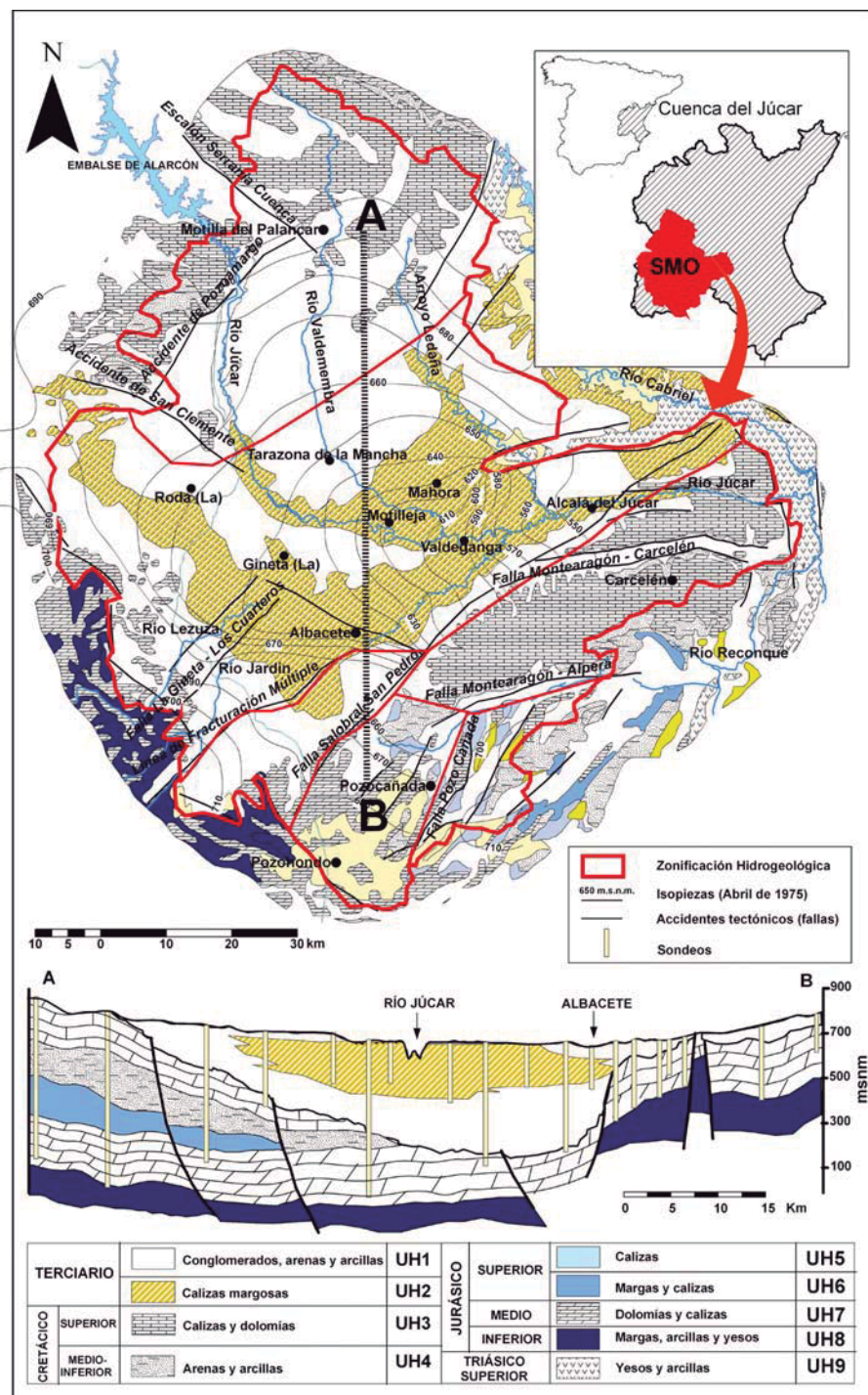
Fig. 1.- Mapa hidrogeológico y corte geológico simplificado del Sistema Mancha Oriental. Isopiezas para abril de 1975 (modificado de Sanz, 2005).
