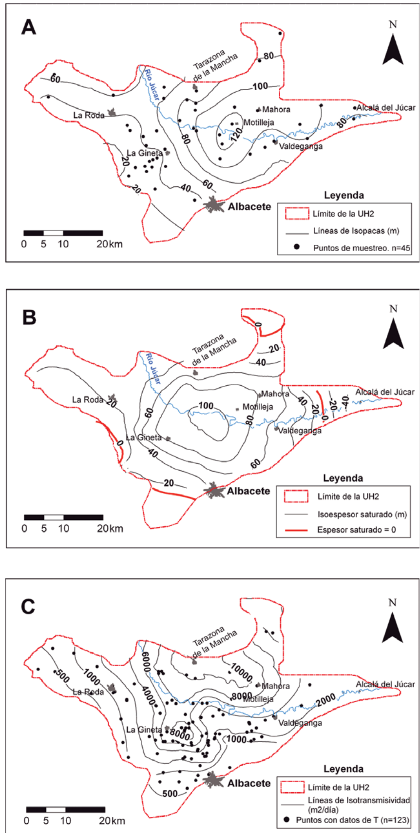
Fig. 2.- Mapas de A) isopacas, B) espesor saturado, y C) isotransmisividad de la Unidad Hidrogeológica 2 (UH2).
