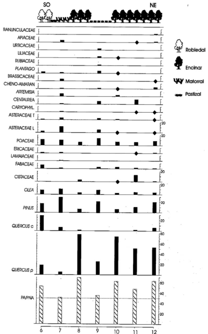
Fig. 3.- Transect TL2. (Dorado Valiño, 1993).
