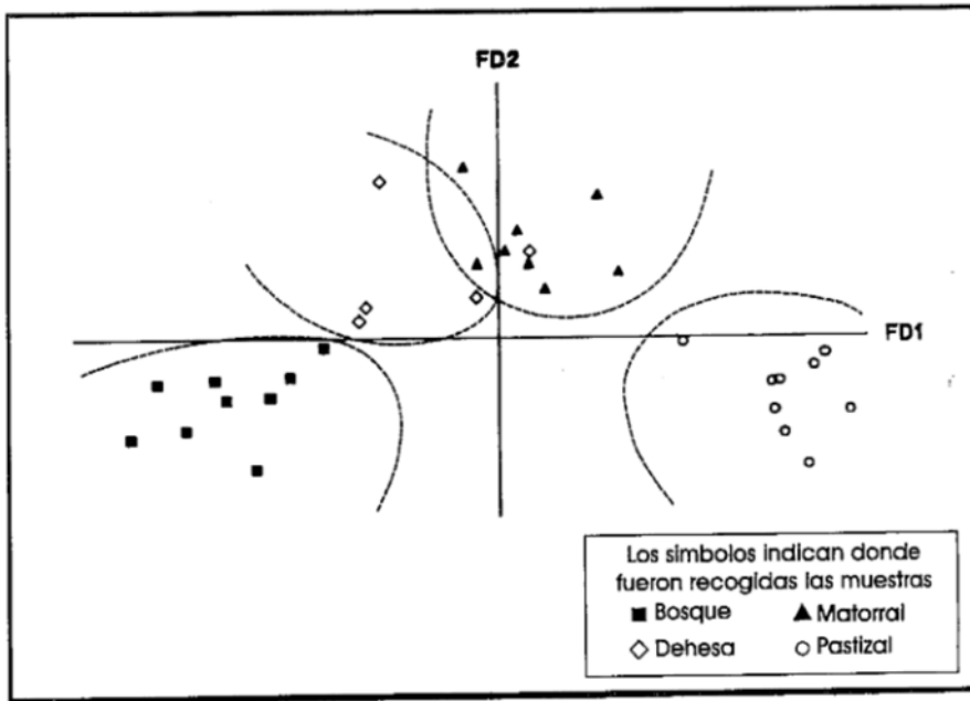
Fig. 4.- Representación de los espectros polínicos en el plano de discriminación F1 X F2 (Dorado Valiño, 1993)
