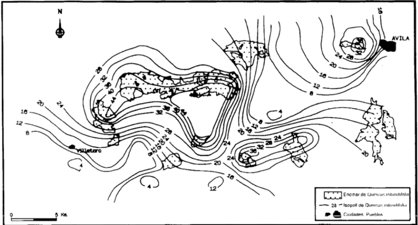
Fig. 2.- Curvas isopoll de Quercus rotundifolia . (Dorado Valiño, 1993).
