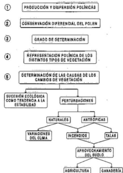
Fig.1.-Consideraciones previas a la interpretación de un Diagrama Polínico.
