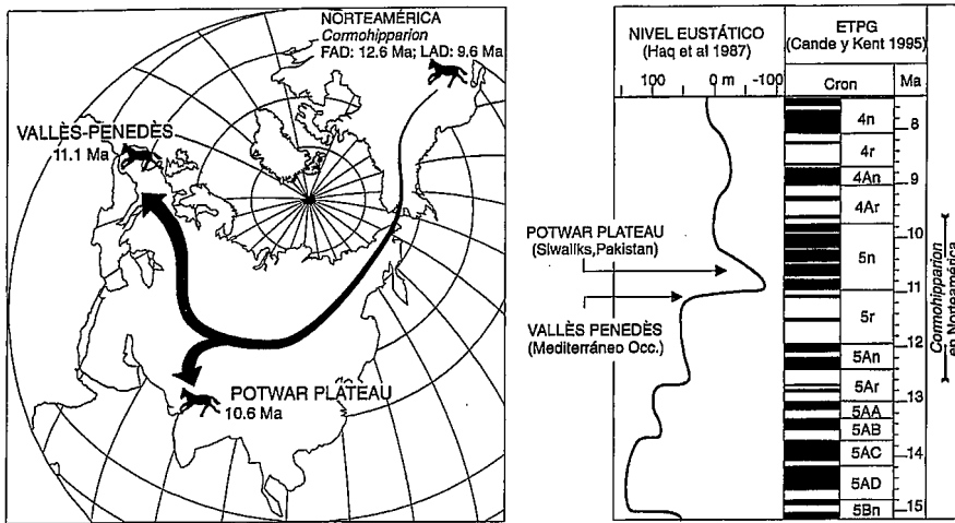
Fig. 2.- La dispersión de Hipparion en el Viejo Mundo implicó una vía temporal de comunicación entre Norteamérica y Asia a través del estrecho de Bering. La datación de la aparición de Hipparion en el Mediterráneo en 11.1 Ma sugiere que la apertura del paso de Bering fue consecuencia de una pronunciada bajada eustática registrada cerca del límite Serravallense/Tortonense (Haq et al, 1987).
