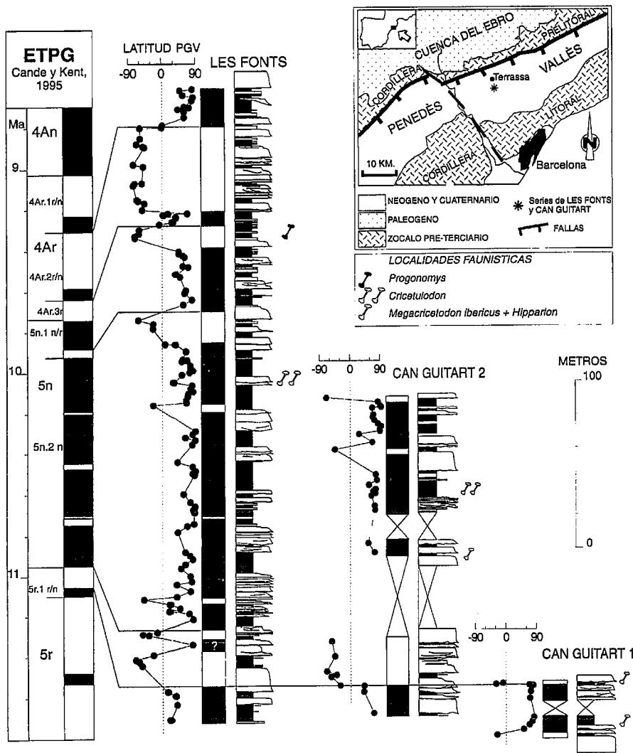
Fig. 1.- Secuencia de polaridad magnética de las series de Les Fonts y Can Guitart 1 y 2 (Cuenca del Vallès-Penedès) y correlación con la ETPG. Los puntos indican la latitud del Polo Geomagnético Virtual media para cada estación.
