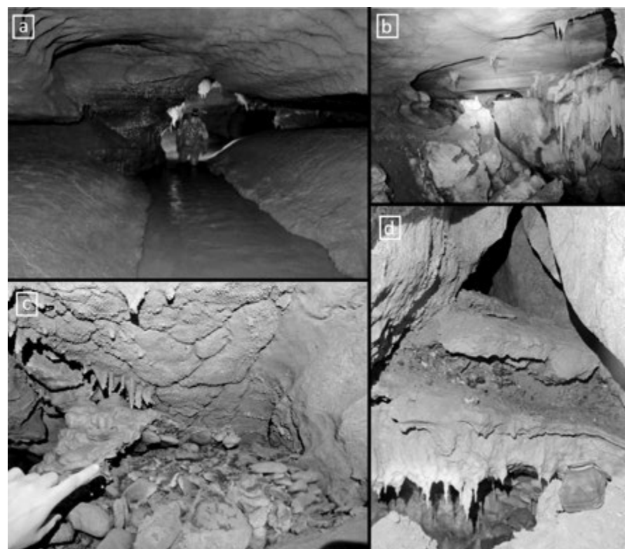
Fig. 2.- a) El tránsito epifreático del río Urtxume donde se observa un canal de techo. b) Galería con canales de techo y la base desmantelada de NC4. c) Canales anastomosados en los planos de techo asociados con los conglomerados alóctonos. d) Conducto meandriforme que conecta diferentes niveles de cuevas, parcialmente relleno de conglomerados alóctonos. Ver figura en color en la Web.
