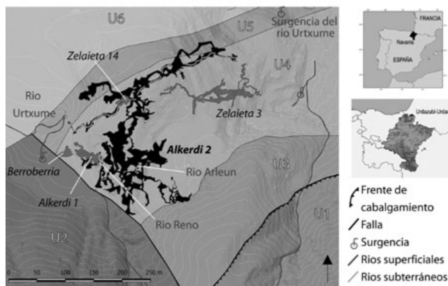
Fig. 1.- Localización, contexto geológico y desarrollo del macizo kárstico Alkerdi-Zelaieta. U1: Esquistos paleozoicos; U2: Areniscas rojas triásicas; U3: Areniscas albienses; U4: Calizas rojas con rudistas; U5: Calcarenitic limestone; U6: Calcareous Flysch. Ver figura en color en la web.
