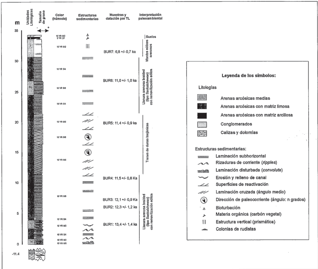
Fig. 2- Columna sedimentológica, localización de las muestras con la datación por luminiscencia, e interpretación paleoambiental basada en las estructuras sedimentarias. Legenda de los símbolos y tramas: Litologías; 1, arenas arcóscas medias; 2, arenas arcóscas con matriz limosa; 3, arenas arcóscas con matriz arcillosa; 4, conglomerados; 5, calizas y dolomías. Estructuras sedimentarias; a, laminación subhorizontal; b, rizaduras de corriente (ripples); c, laminación disturbada (convolute); d, erosión y relleno del canal; e, superficies de reactivación; f, laminación cruzada (ángulo medio); g, dirección de paleocorriente (ángulo, n grados); h, bioturbación; i, materia orgánica (carbón vegetal); j, estructura vertical (prismática); k, colonias de rudistas.
