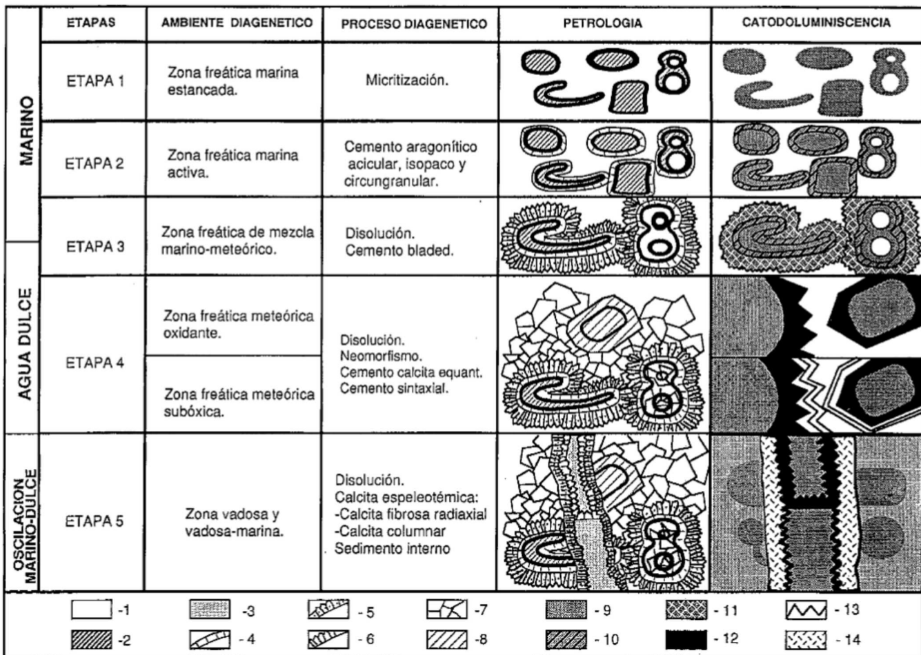
Fig. 2 — Diagrama ilustrando las diferentes etapas diagenéticas y sus modelos de petrología y catodoluminiscencia: 1- Porosidad, 2- Bioclastos, 3- Sedimento interno, 4- Cemento acicular, 5- Cemento bladed y radiaxial rico en inclusiones, 6- Cemento bladed o columnar libre de inclusiones, 7- Cemento equant, 8- Cemento syntaxial. Los números del 9 al 14 se refieren al color de catodoluminiscencia: 9- Dull, 10- Dull con parches no luminiscentes, 11- Dull con parches brillantes, 12- No luminiscente, 13- Brillante zonado, 14- Brillante con parches dull.
