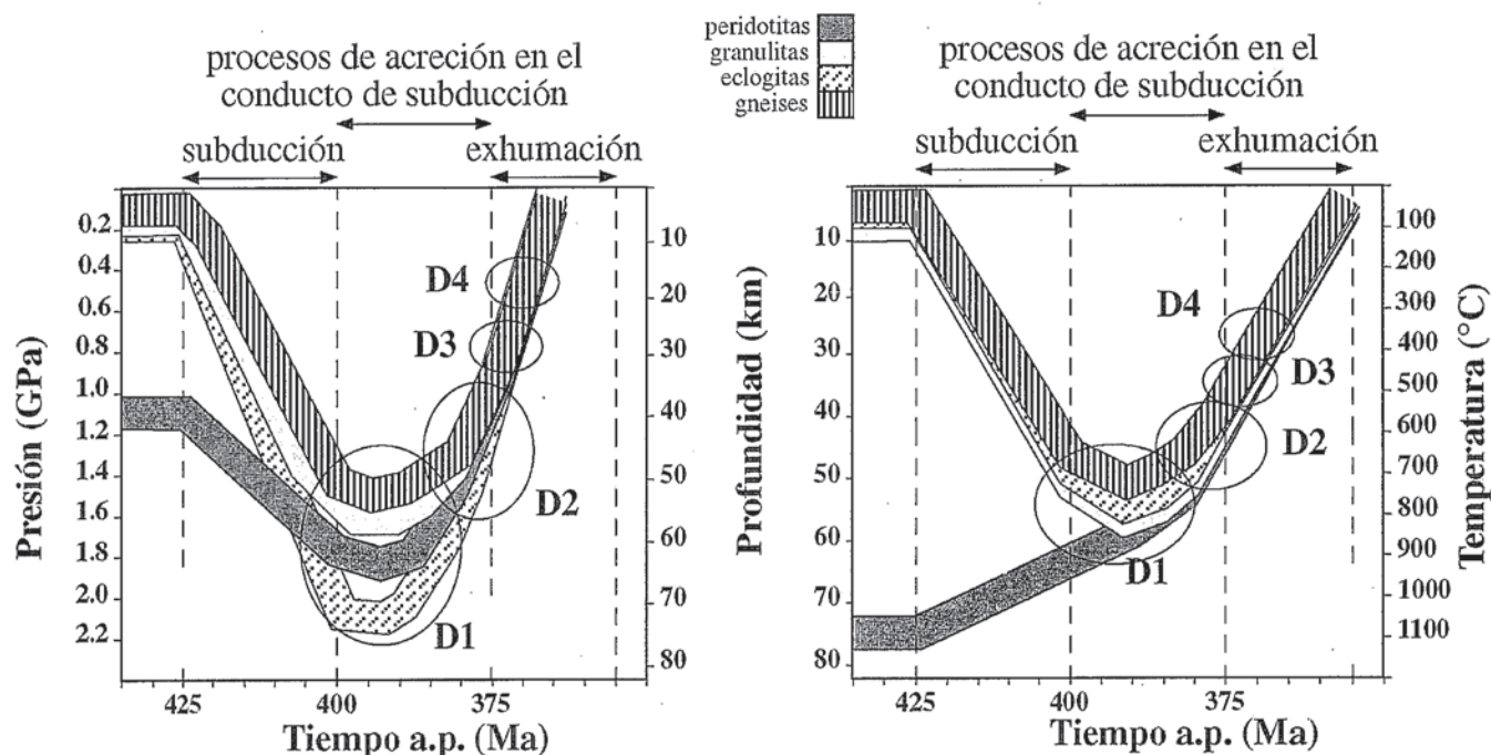
Fig. 2.- Reconstrucciones cinemáticas en el marco presión/profundidad y temperatura/tiempo de la evolución de las unidades de alta presión durante los procesos de subducción, acreción tectónica y flujo de retorno forzado en el canal de subducción y la exhumación subsiguiente durante la colisión orogénica. La escala de profundidad corresponde a un modelo litosférico formado por 15 km de rocas de la corteza superficial con una densidad media de 2700 kg/m 3 , 15 km de rocas de la corteza inferior de 2900 kg/m 3 y rocas mantélicas de 3300 kg/m 3 .
