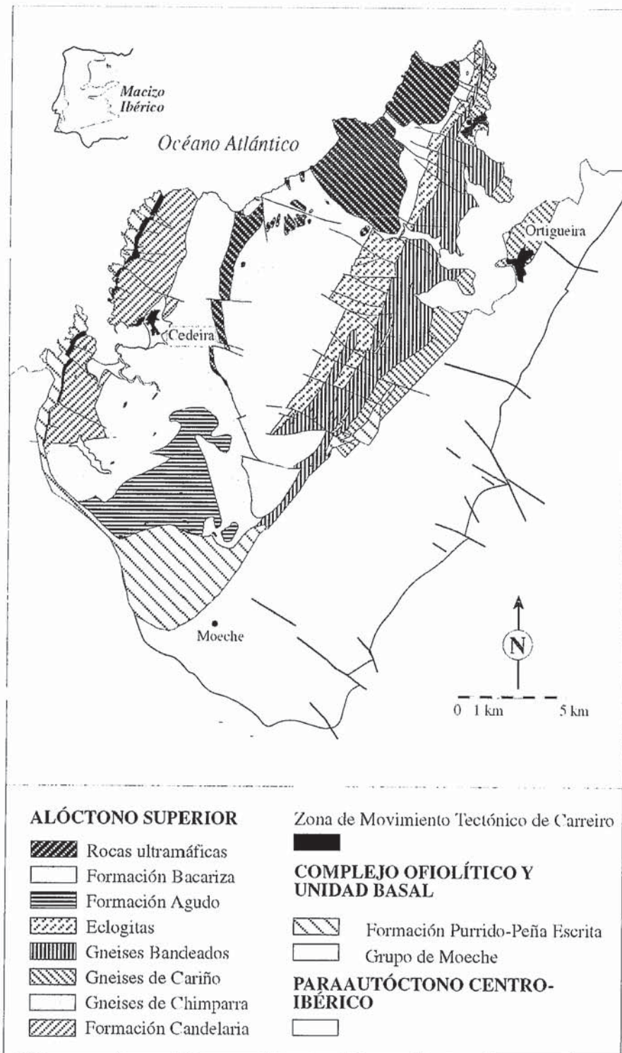
Fig. 1.- Mapa geológico simplificado del Complejo de Cabo Ortegal.
