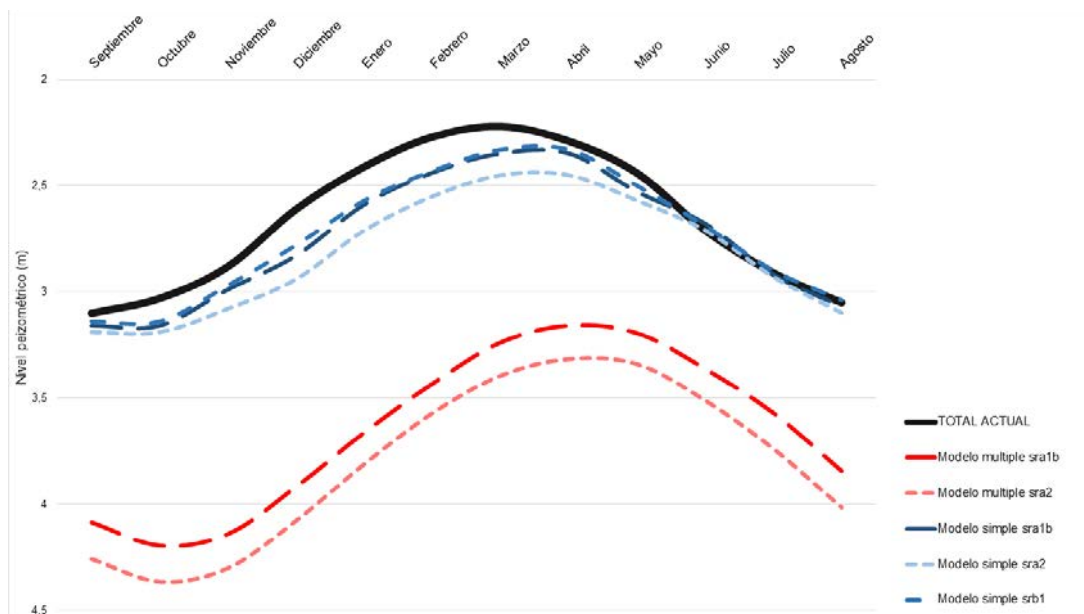
FIGURA 6 COMPARACIÓN ENTRE LOS NIVELES PIEZOMÉTRICOS CORRESPONDIENTE A UN AÑO PROMEDIO EN EL PRESENTE (EN NEGRO) Y LOS PRONÓSTICOS PARA FINALES DEL SIGLO XXI REALIZADOS A PARTIR DEL MODELO ECHAM5
